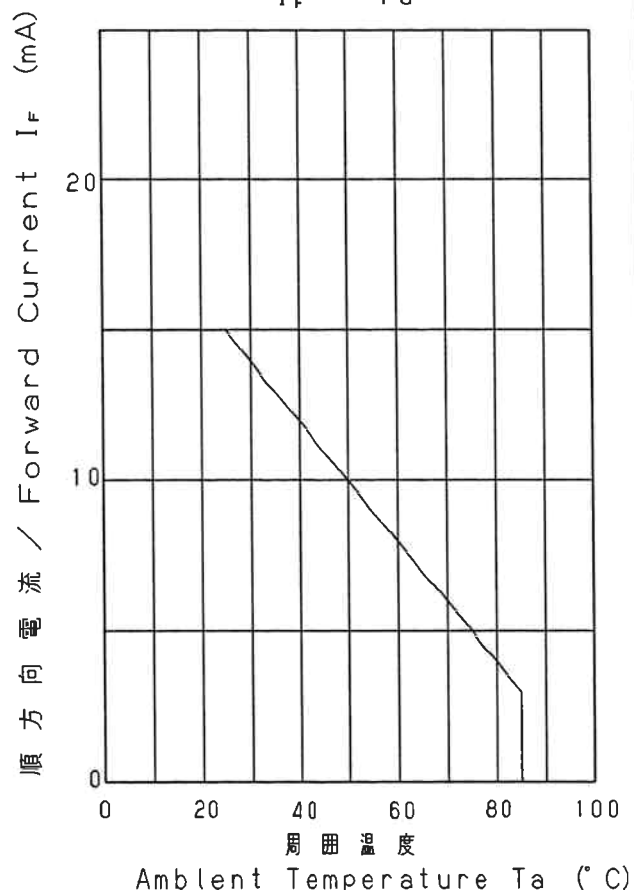
I_F - T_a
