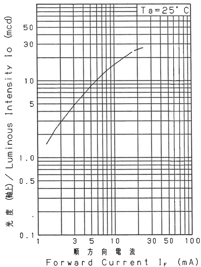
I_0 - I_F
