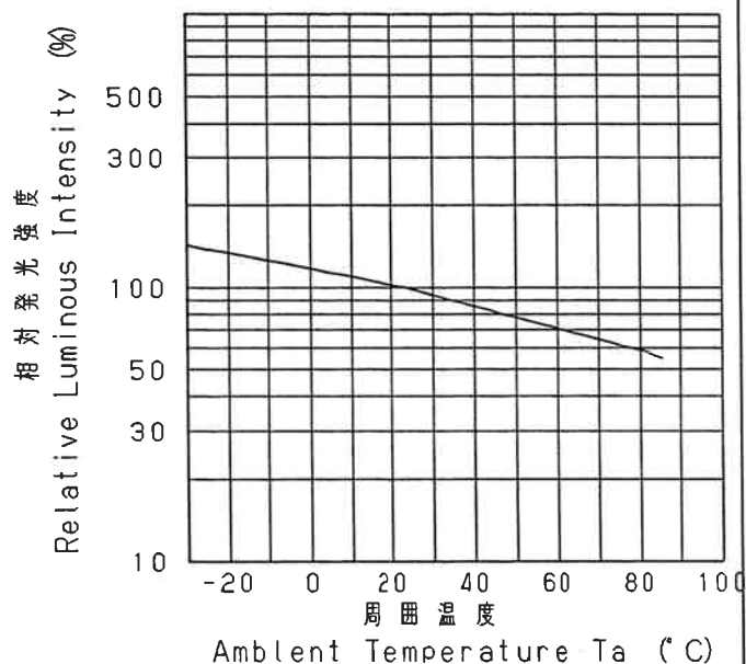
I_0 - T_a
