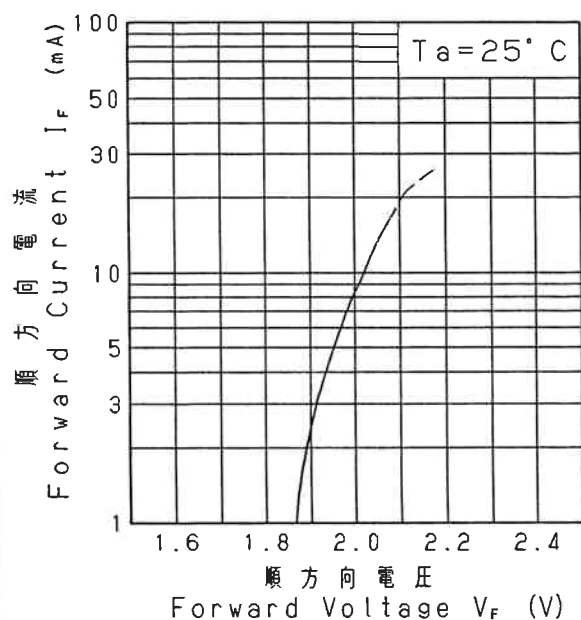
I_F - V_F
