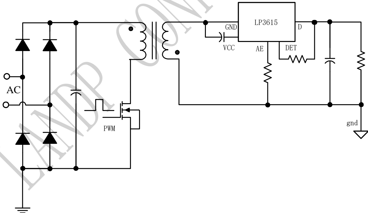
图 1 LP3615 典型应用图
