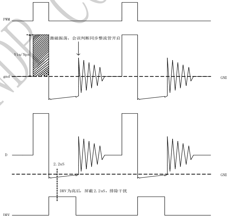
图 4 系统关键节点相对于 LP3615 的 GND 波形
