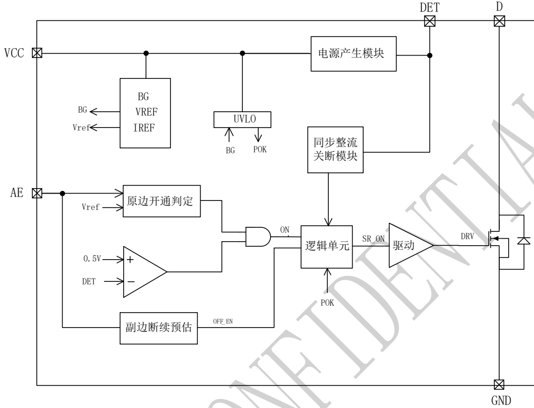
图 3 LP3615 内部框图
