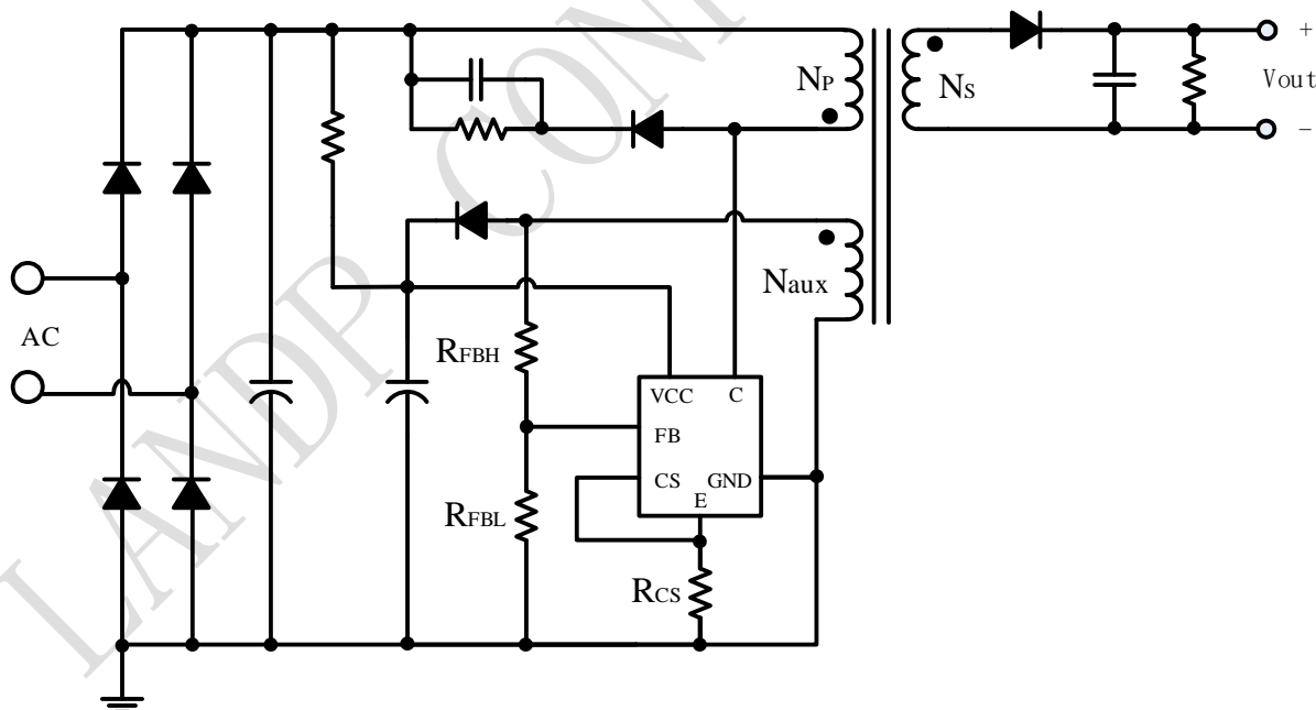
图 1 LP3773 典型应用图
