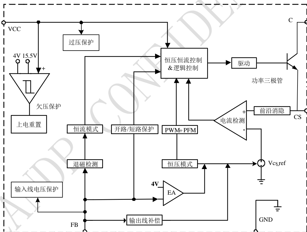
图 3 内部框图
