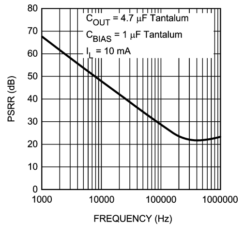
V_{IN} PSRR
