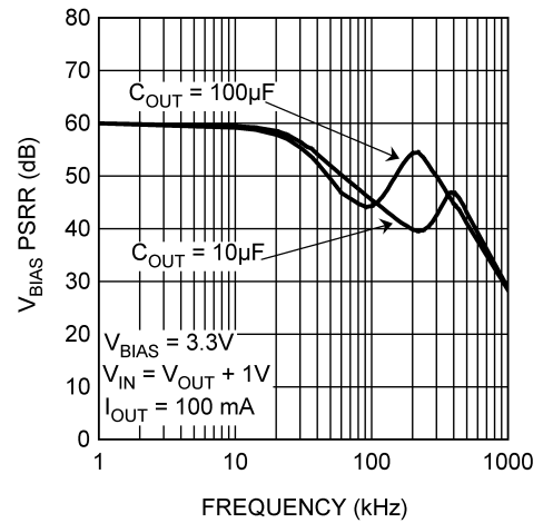
V_{BIAS} PSRR
