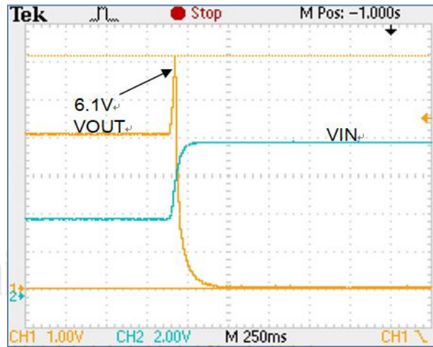
OVP waveform
