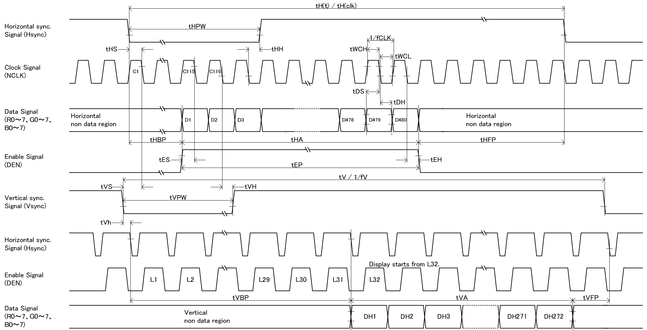
図 2 : 入力信号タイミング波形 Fig.2 : Input signal timing waveform
