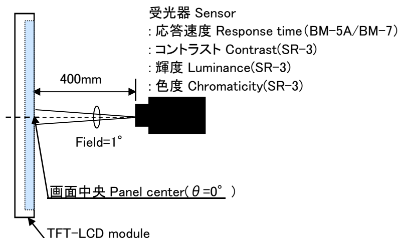
図3-2 コントラスト/輝度/応答速度/色度特性測定方法
