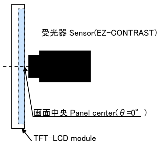
図3-1 視野角特性測定方法
