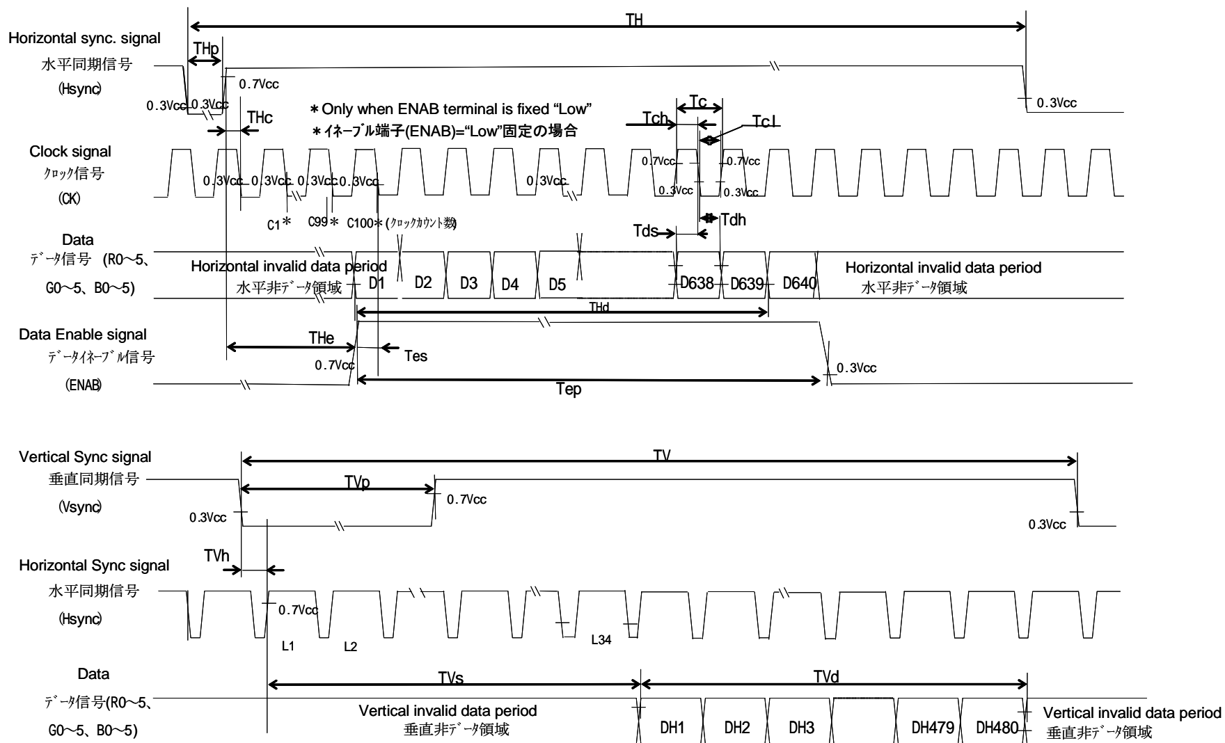
Fig 2. Input signal waveform 図2. 入力信号タイミング
