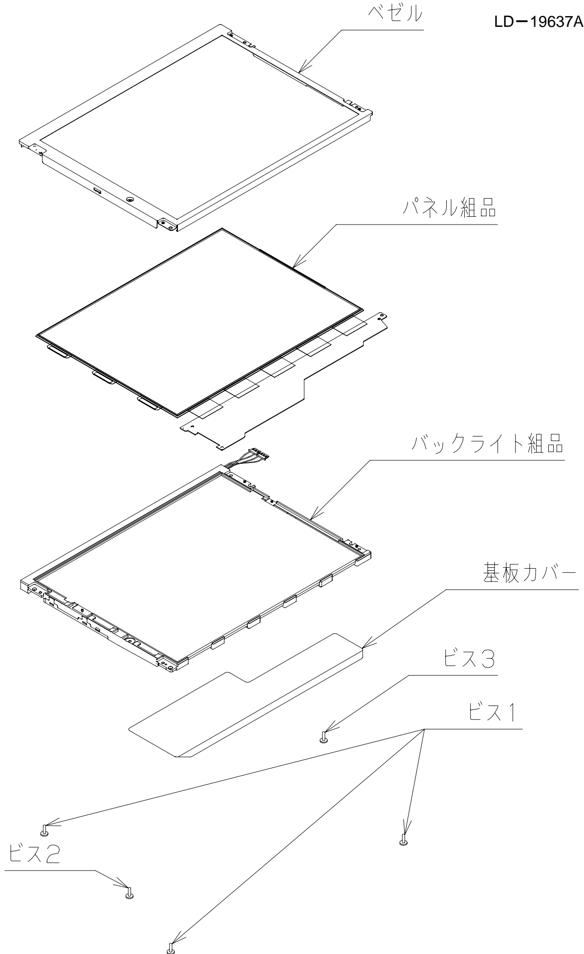
図4 . モジュール組立形態図
