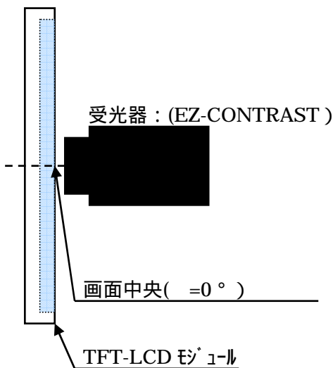
図 2-1 視野角特性測定方法
