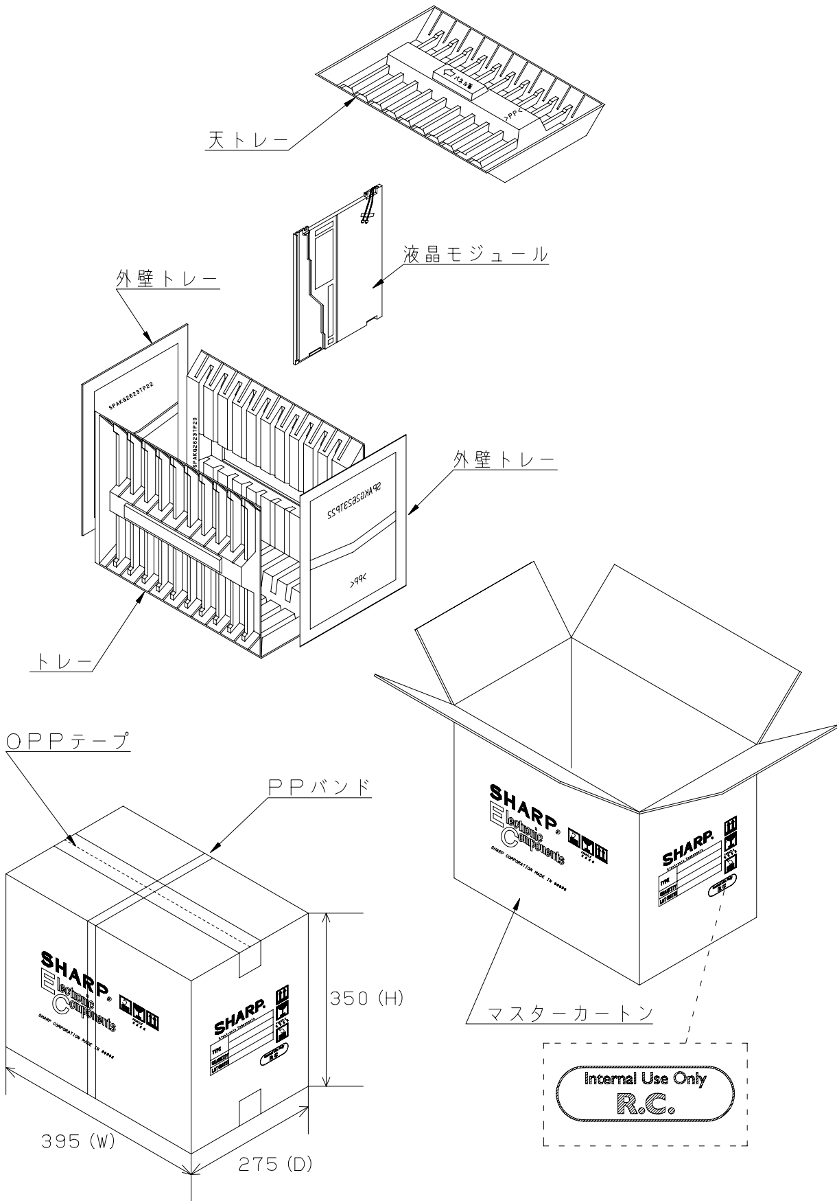
図 3 : 包装形態図
