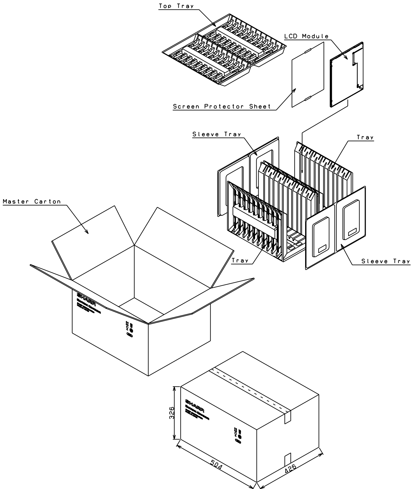
图3. 包装形态图
