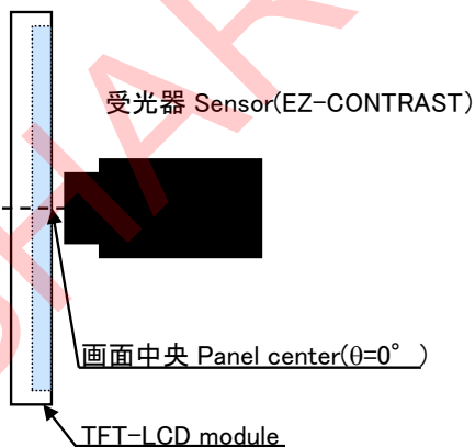
図2-1 視野角特性測定方法
