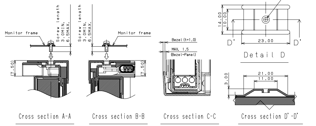
Fig.1:Outline dimensions (LQ190E1LW43)
