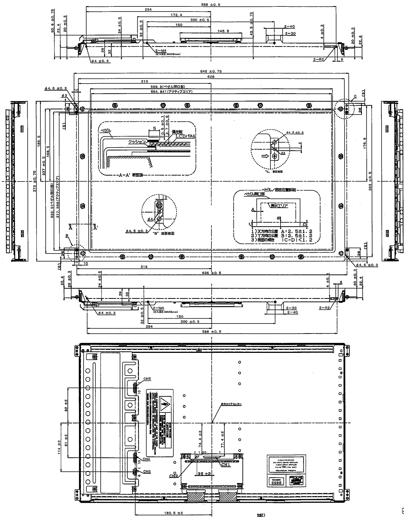
図1. LQ255T3LZ21 TFT-LCDモジュール外形図
