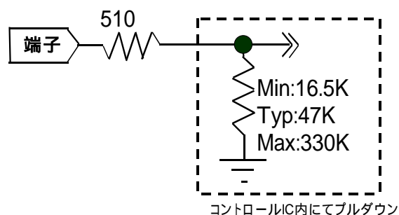
【注3】 端子の等価回路図
