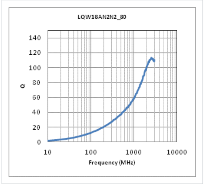
■ Q-周波数特性(代表値)
