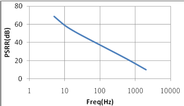
4. PSRR
