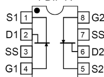
PDIP-A
