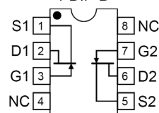
PDIP-B
