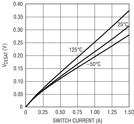
V CESAT
