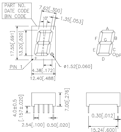
A. LTS-546A/547A
