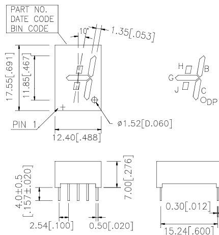
B. LTS-548A/549A
