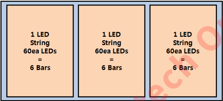
LCD Module
