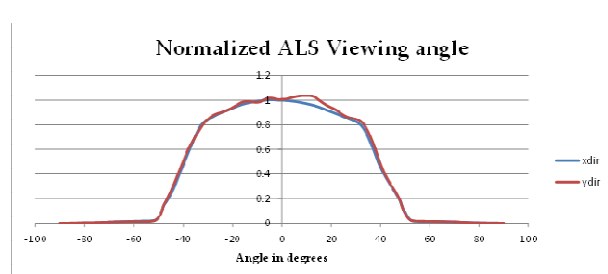
Figure 4.2 ALS Sensitivity vs. Angular of Incidence
