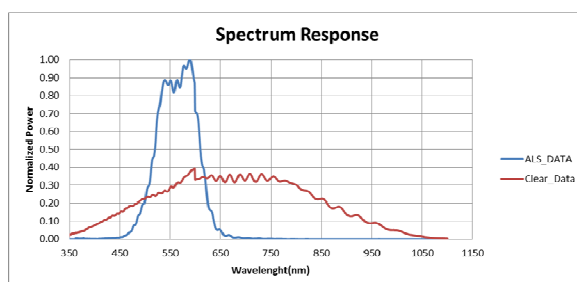
Figure 4.1 : Spectral response for ALS
