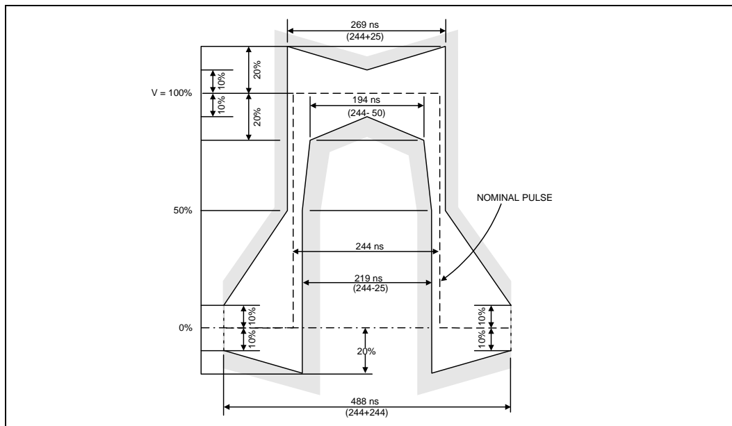
Figure 20. E1, G.703 Mask Templates
