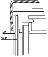
SECTION YY-YY SCALE 5:1
