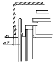
SECTION YY-YY SCALE 5:1
