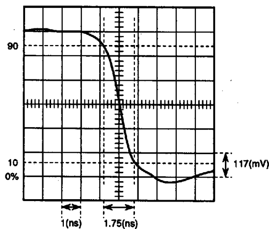
M52328SP FALL
