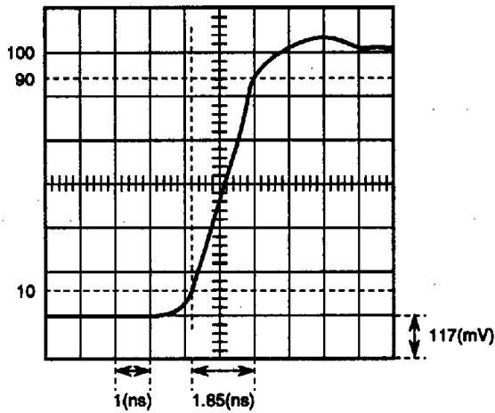
M52328SP RISE
