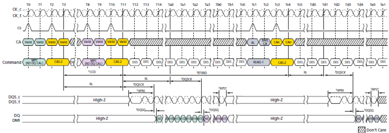
Figure 119. Read DQ Calibration Training Timing: Read DQ Calibration to Read DQ Calibration/Read
