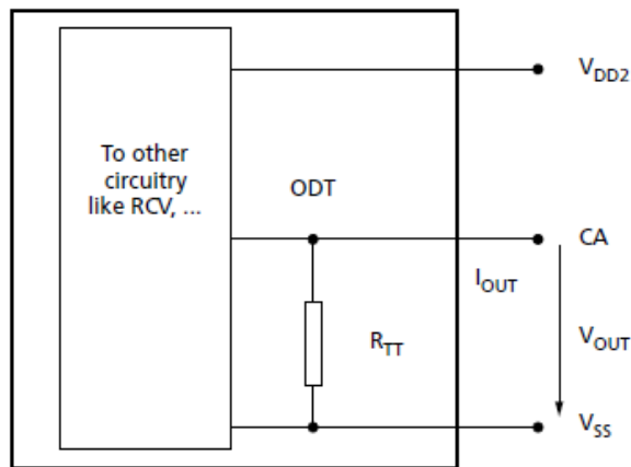
ODT for CA
