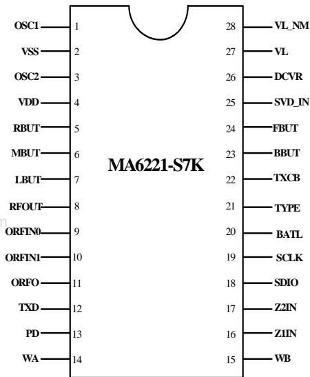
SOP28
