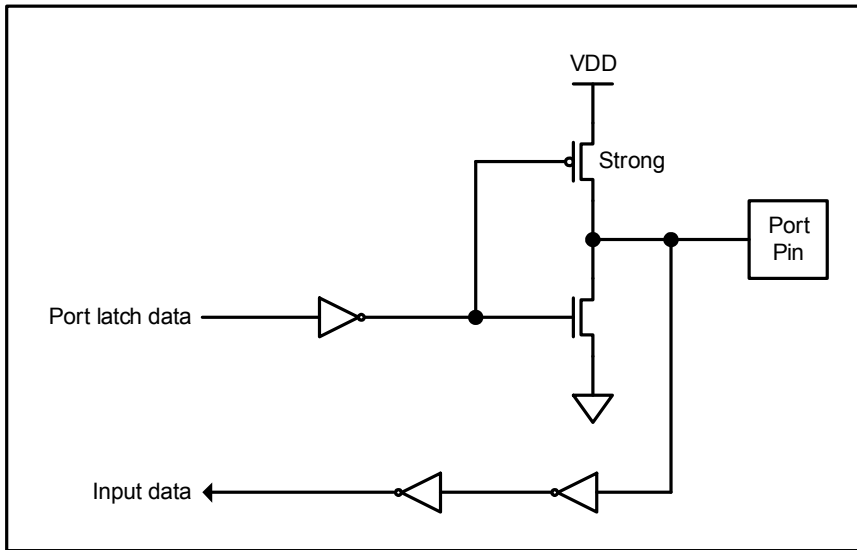
图 10-2 推挽输出
