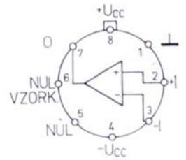
Соединение выводов (вид снизу)
