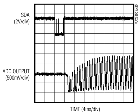
SOFT-START ADC
