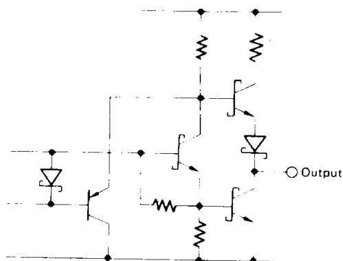
Fig. 5 – MB 7132 OUTPUT
