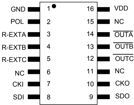
MBI6021GP 正面
