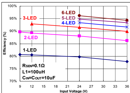
Fig 10. I_{OUT}=1A
