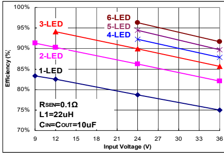
Fig 4. I_{OUT}=1A
