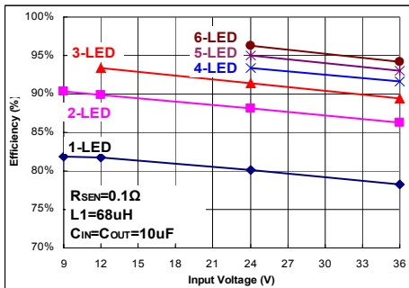
Fig 7. I_{OUT}=1A
