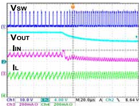
Fig. 83. Short-circuit protection
