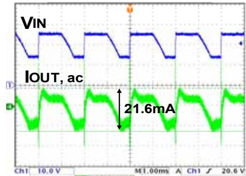
Fig 70. L1=68\mu H
