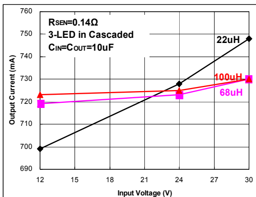
Fig 26. I_{OUT}=715 mA
