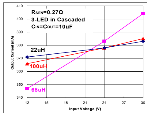
Fig 27. I_{OUT}=370 mA
