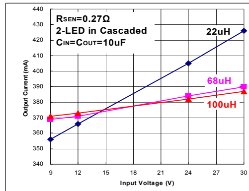
Fig 25. I_{OUT}=370 mA
