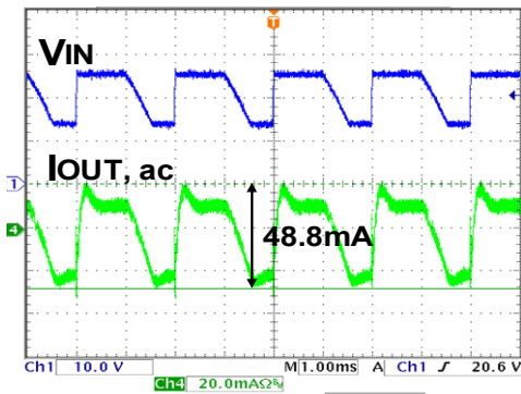
Fig 48. L1=22\mu H
