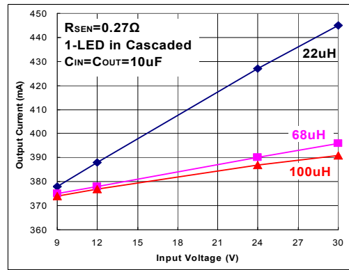
Fig 23. I_{OUT}=370 mA
