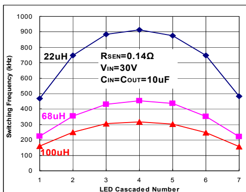
Fig 44. I_{OUT}=715\text{ mA}
