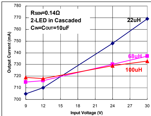
Fig 24. I_{OUT}=715 mA
