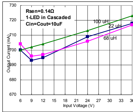
I_{OUT}=700mA Fig. 32
