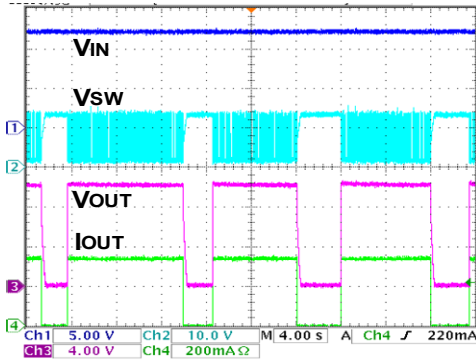
Fig. 73 Thermal protection
