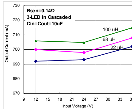
I_{OUT}=700mA Fig. 38
