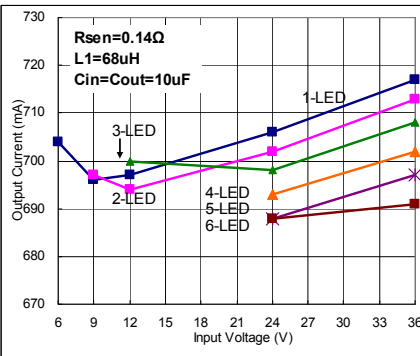
I_{OUT}=700mA Fig. 26
