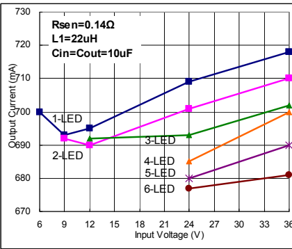
I_{OUT}=700mA Fig. 23
