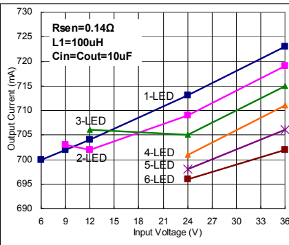
I_{OUT}=700mA Fig. 29
