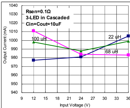
I_{OUT}=1A Fig. 37
