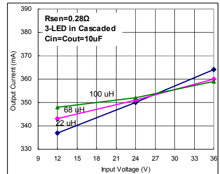
I_{OUT}=350mA Fig. 39
