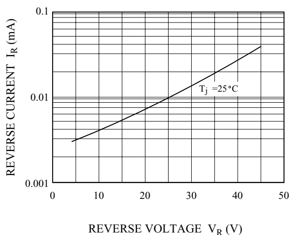
I_R - V_R
