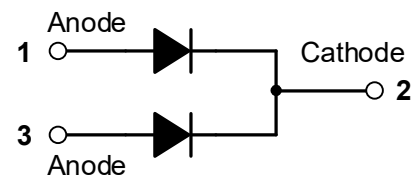
TO-263AB(D²PAK)
