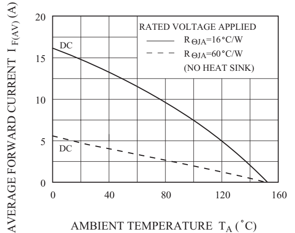
I_F - T_A
