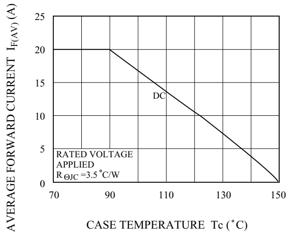
I_F - T_c
