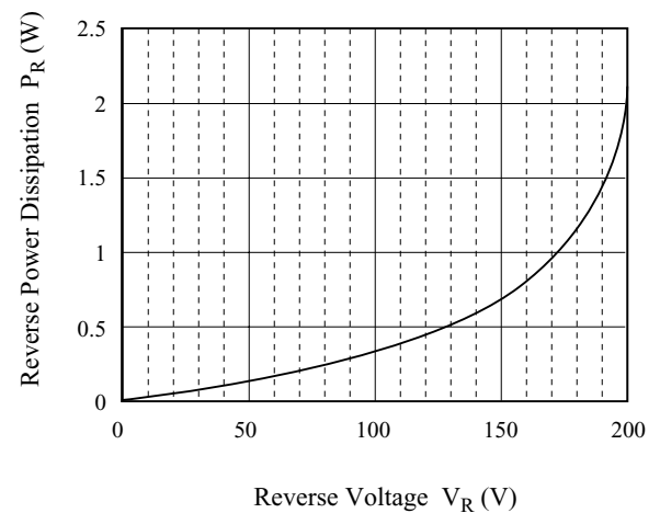
P_R - V_R
