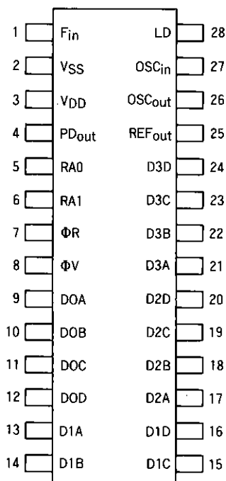
ピン配置図 (Pサフィックス)
