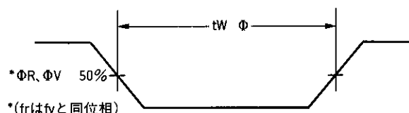
図4 スイッチング波形
