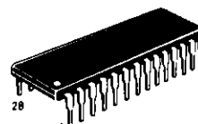
P サフィックス プラスチック DIL パッケージ ケース710
