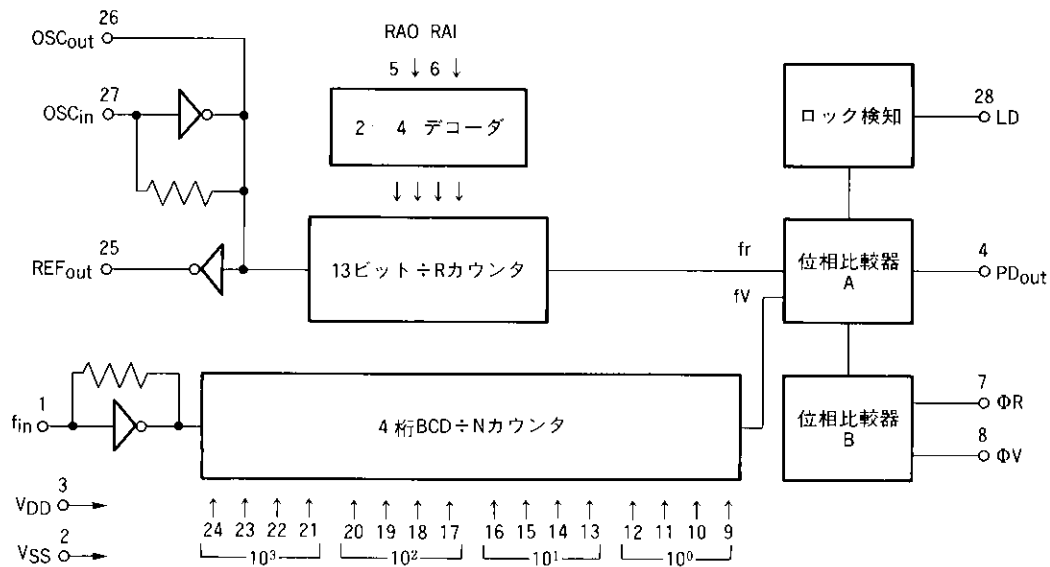
ブロック図
