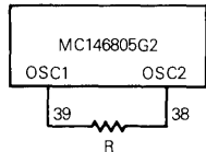
(d) RC Oscillator Connection
