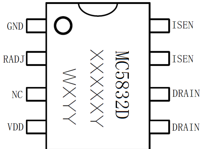
图 2 芯片引脚图
