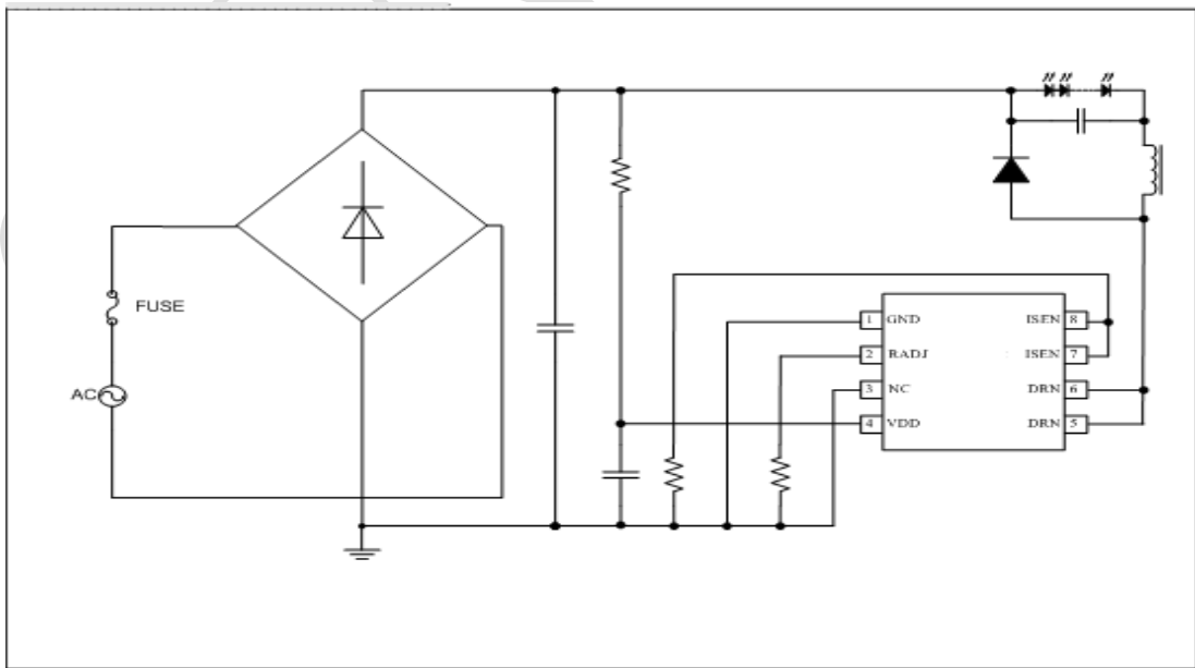
图 1 MC5832D 典型应用图
