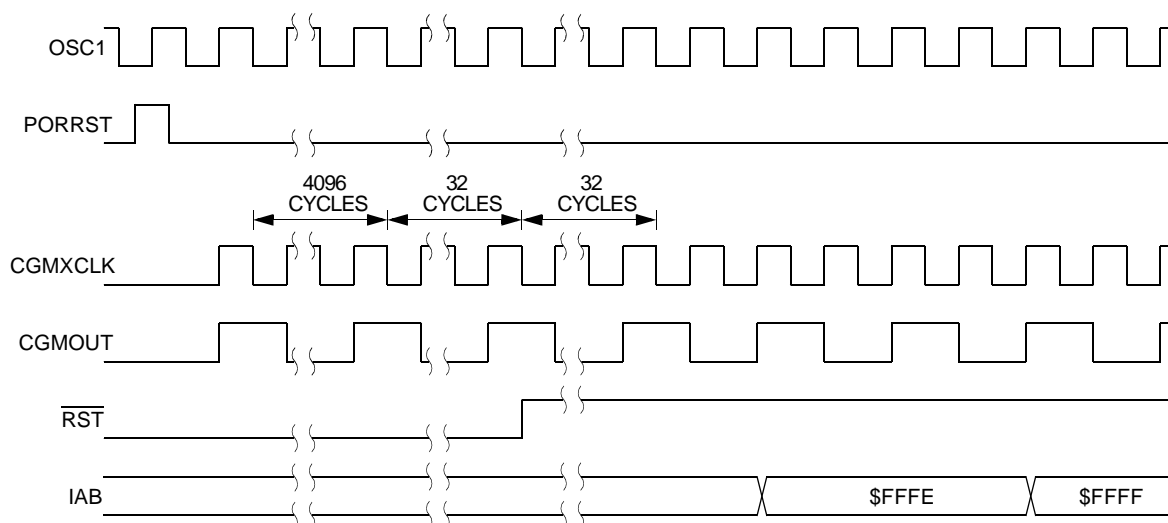
Figure 8-6. POR Recovery
