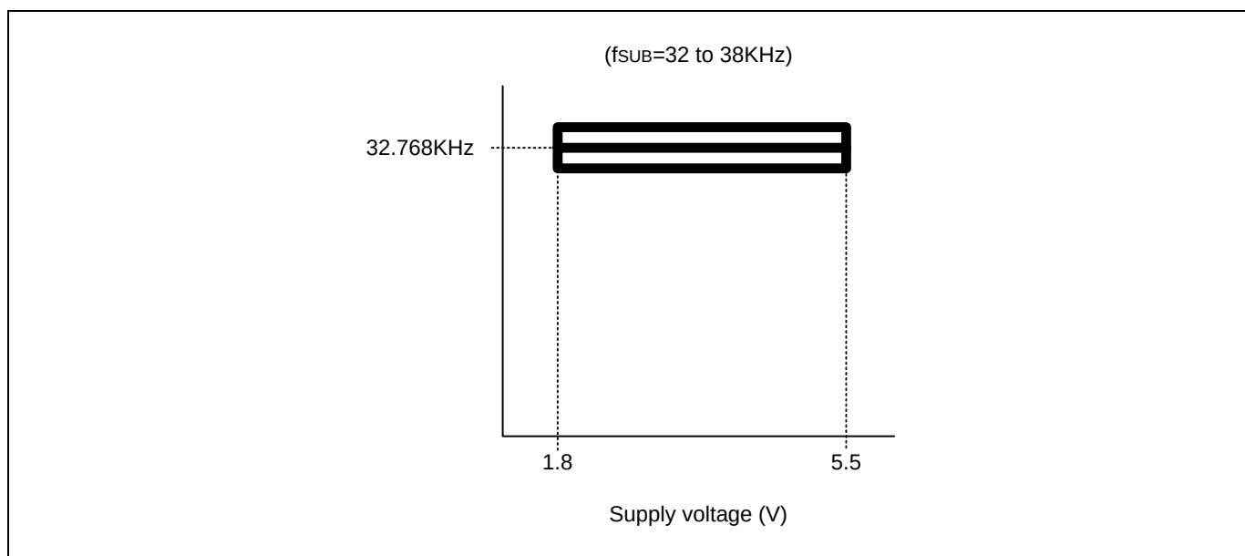
Figure 7.10 Operating Voltage Range (Sub OSC)
