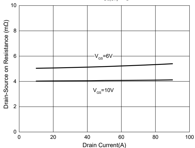
Fig. 7 - R_{DS(ON)} - I_D
