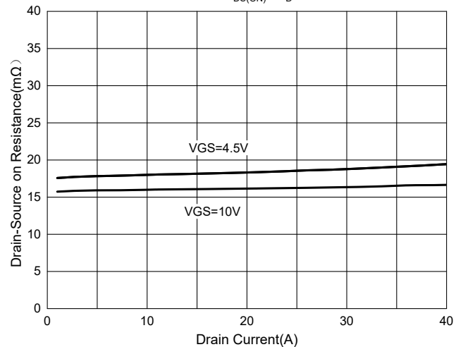
Fig. 4 - R_{DS(ON)} - I_D
