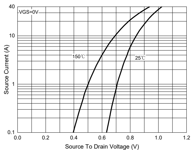
Fig.9 - I_S - V_{SD}
