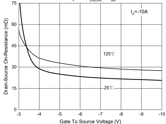
Fig. 5 - R_{DS(ON)} - V_{GS}
