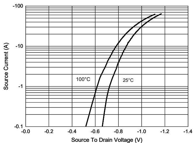
Fig. 7 - I_S - V_{SD}
