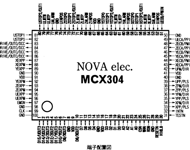
端子配置図
