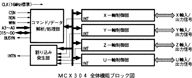
MCX304 全体機能ブロック図
