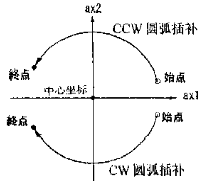
图 2.19 CW/CCW 圆弧插补
