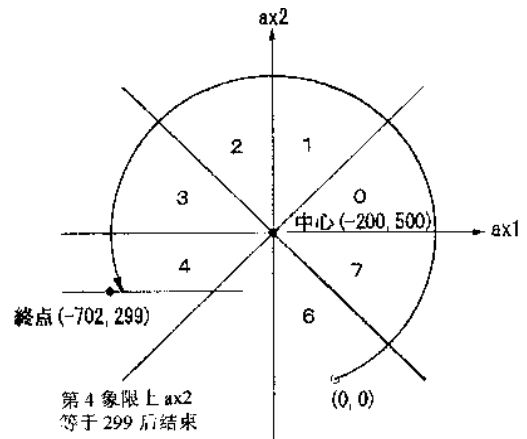
图 2.23 圆弧插补结束判断例子
