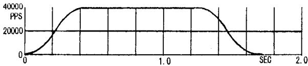
输出脉冲 P=50000
