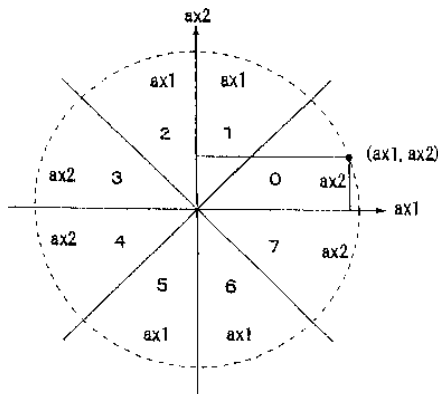
图 2.20 圆弧插补算法的 0~7 象限和短轴
