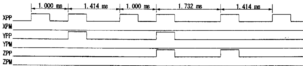
图 2.28 3 轴插补固定线速的例子(线速度:1000PPS)
