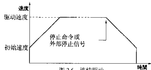
图 2.6 连续驱动
