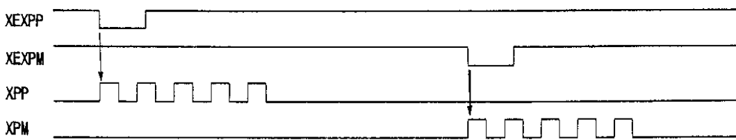
图 2.32 根据外部操作信号输出脉冲 5 的定量驱动例子
