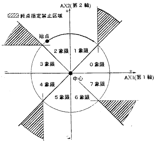
CW 圆弧插补
