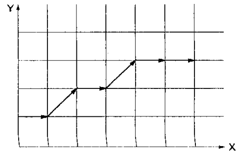
图 2.26 2 轴插补例子
