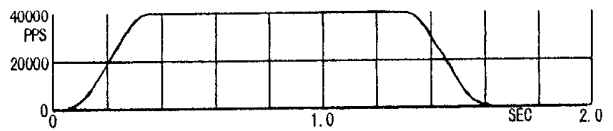
输出脉冲 P=50000
