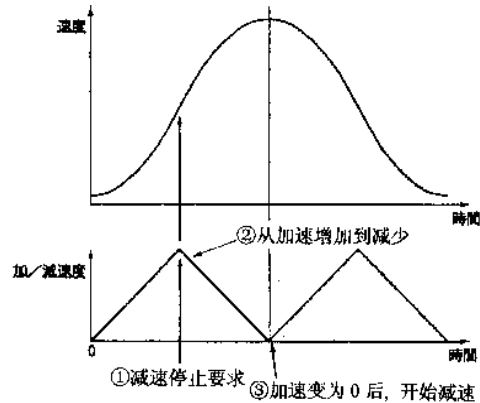
图 2.11 在 S 曲线加/减速的线性加速中减速停止
